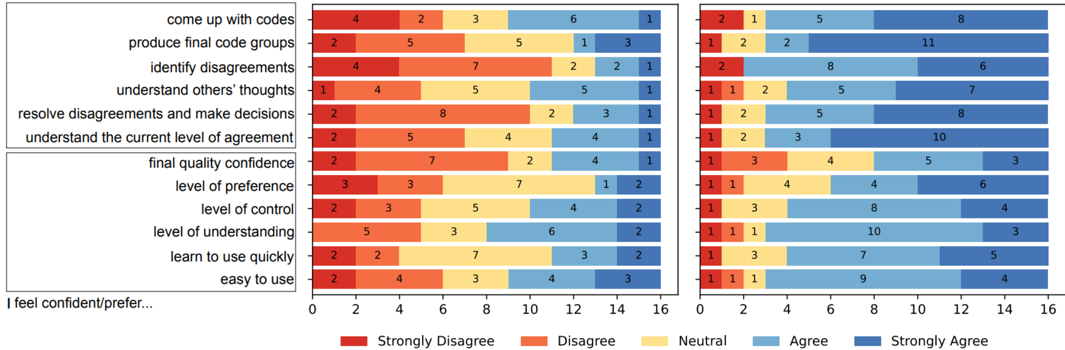
Atlas.ti Web
