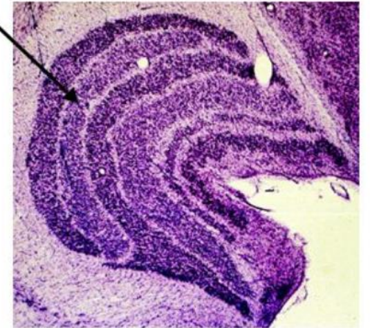
Thalamus (LGN)
